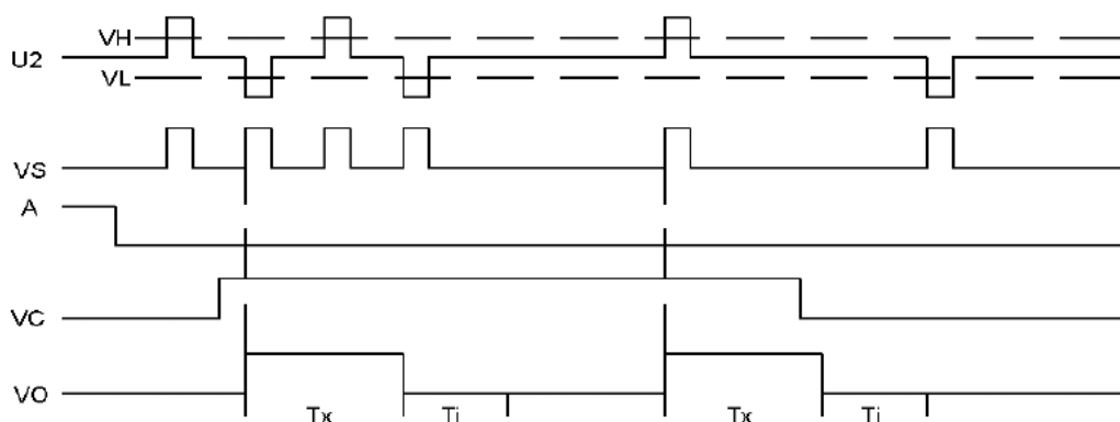
图 3 不可重复触发方式波形
