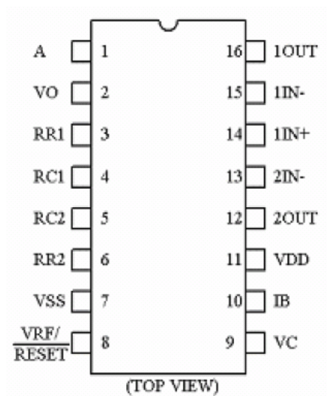
图 2 脚位图
