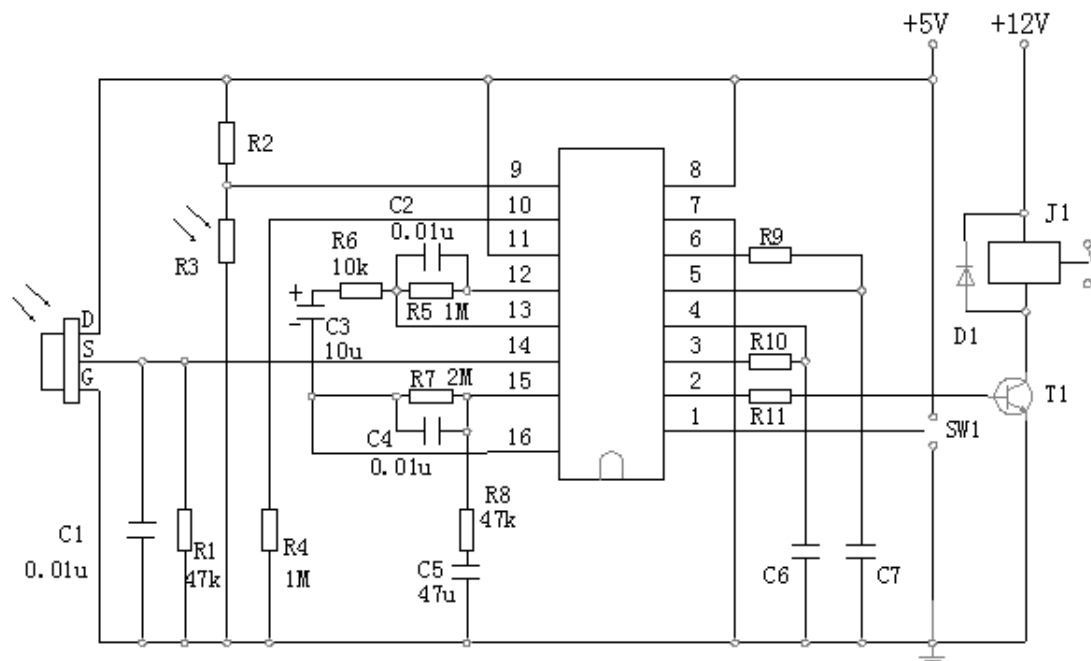
图5 BISS0001典型应用图
