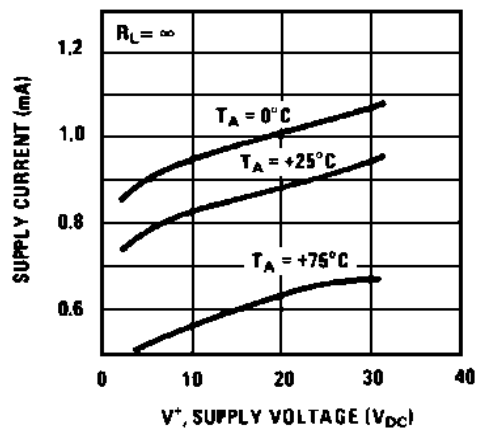
电源电流
