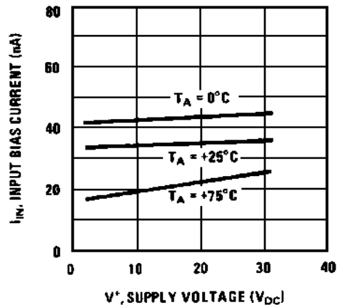
输入电流
